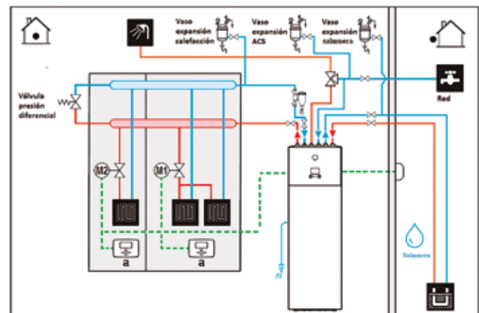
Ejemplo Daikin Altherma GEO con depósito integrado para ACS y suelo radiante
